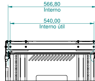
SEÇÃO C-C
