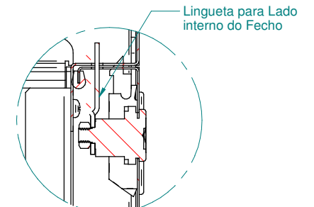
DETALHE D
