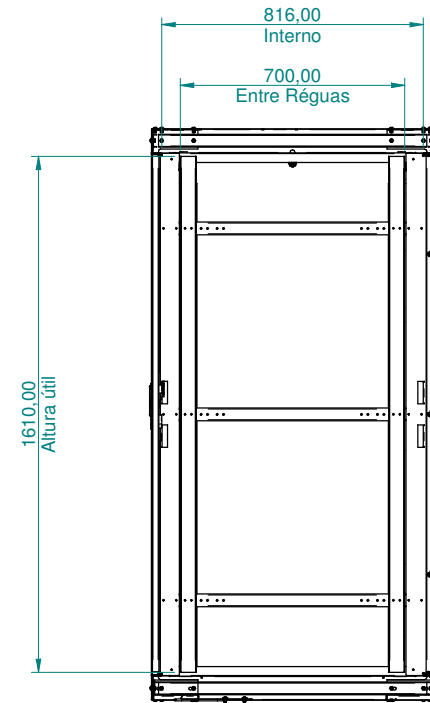
SEÇÃO B-B
